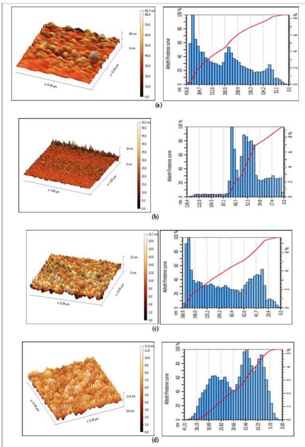
Figure (2): AFM images of; (a)- pure \text{SnO}_2 , (b)- \text{SnO}_2 : 1% Fe, (c)- \text{SnO}_2 : 3 % Fe and (d)- \text{SnO}_2 : 5 % Fe.
