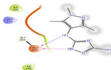
(B) 1,2,4-triazol-3-amine,5-(1,3,5-trimethyl-4-pyrazolyl)
